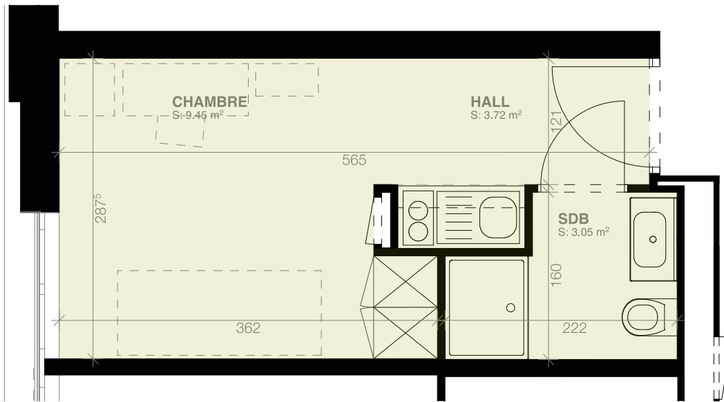
plan appartement typologie 1 appartement: 1 pièce
