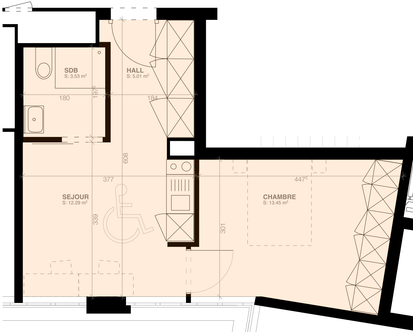
plan typologie 7 appartement PMR: 2 pièces
