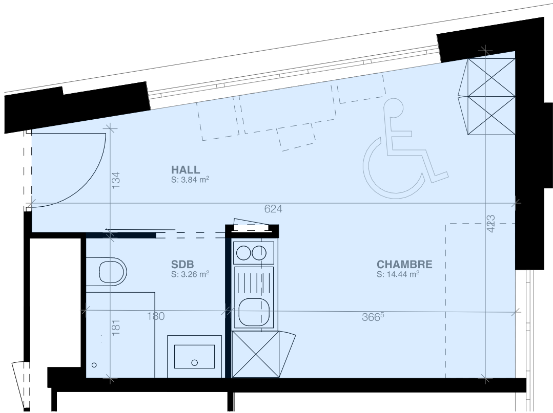
plan appartement typologie 2 appartement PMR: 1 pièce
