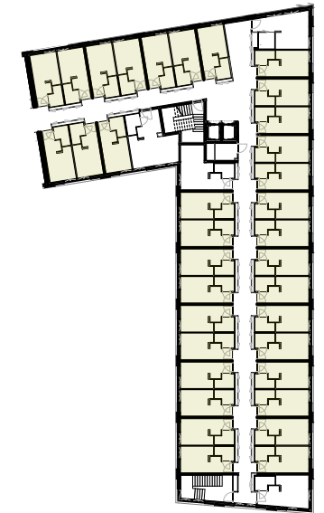
bâtiment L3 étages 1, 2, 3 et 4
