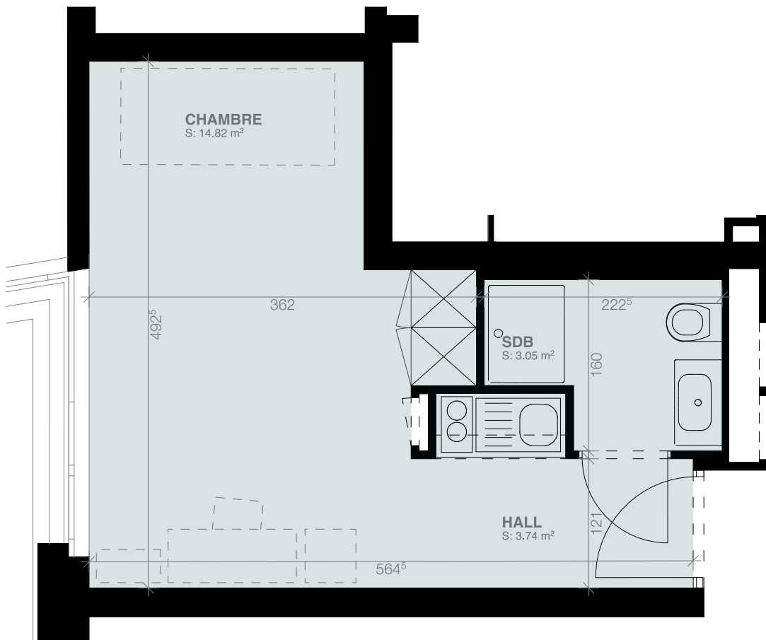
plan appartement typologie 4 appartement:
